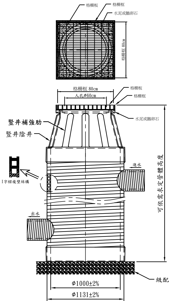
MHS1000X陰井示意圖
