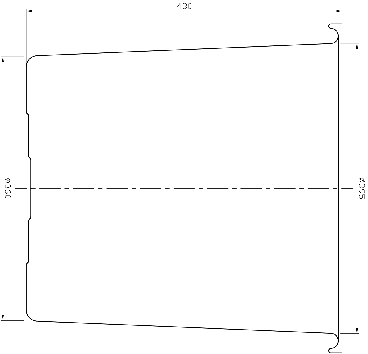
規格 M-47 成品圖
